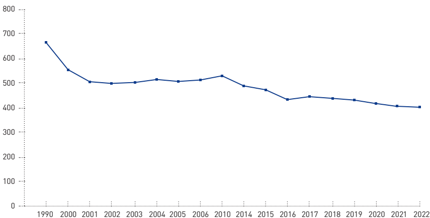
CO 2 -Netto-Emissionen Zementherstellung (kg CO 2 /t)
